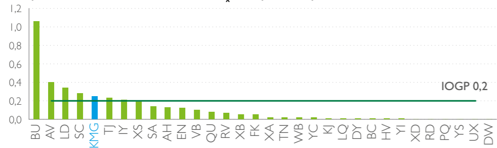
Өндірілген КСШ 1 000 т.м.б. шаққанда NO x шығарындылары, 2018 ж.
